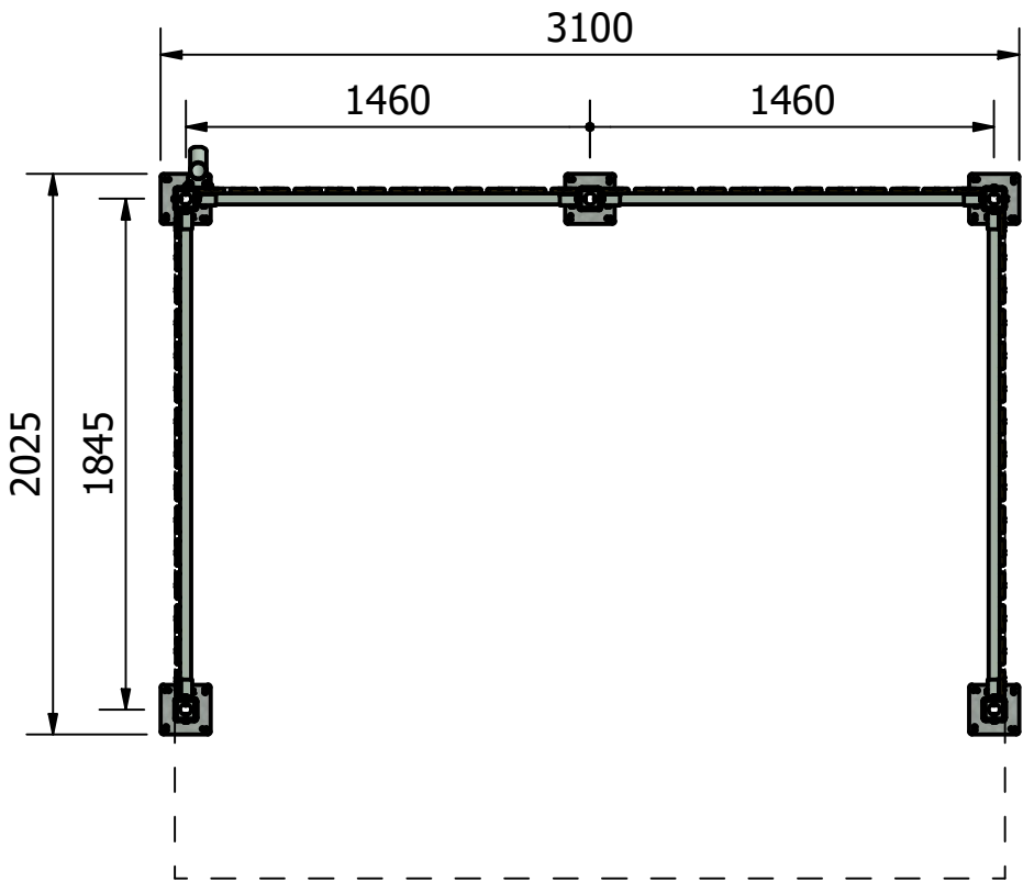
A-A ( 1 : 30 )
